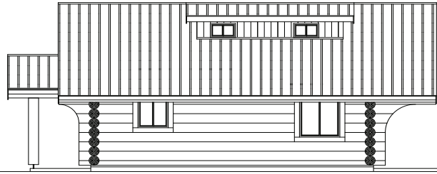
right elevation
