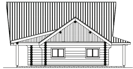
right elevation
