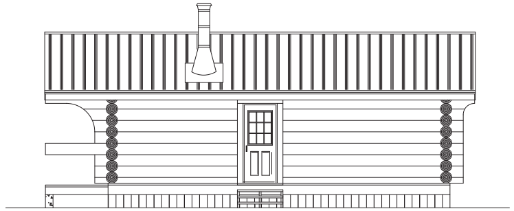
right elevation
